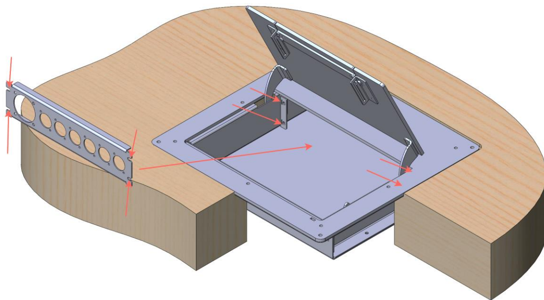
Рис. 3. Установка панели в бок лючка
