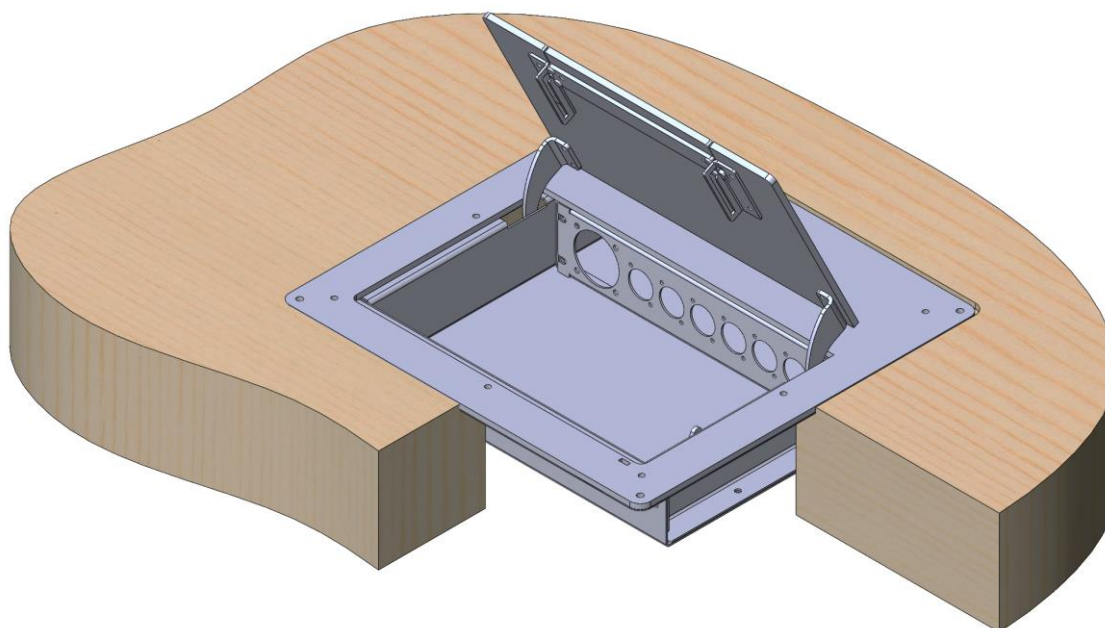
Рис. 4 Лючок с установленной панелью
