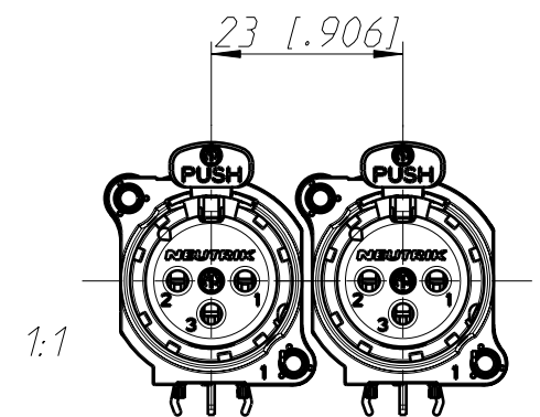
min. Einbauabstand min assembling distance
