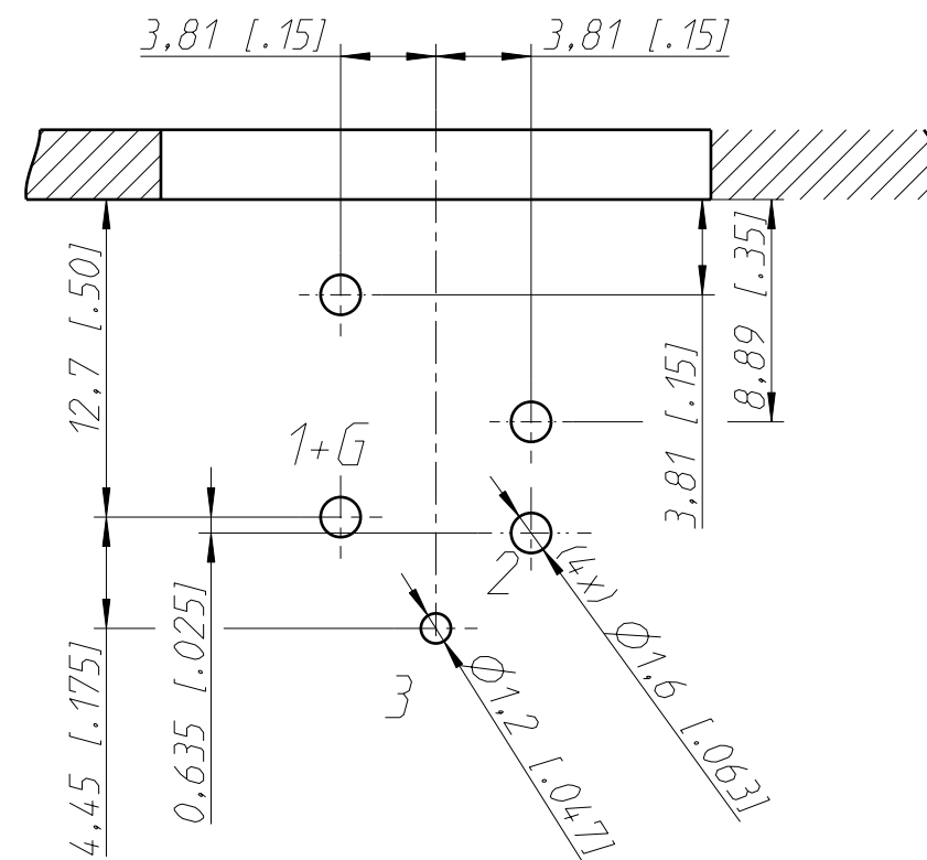
Print-Bohrplan (Bestückungsseite) PCB-Layer (component side)
