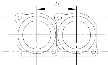
Минимальное расстояние Min assembling distance
