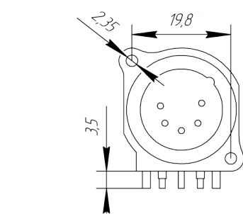
Минимальное расстояние Min assembling distance
