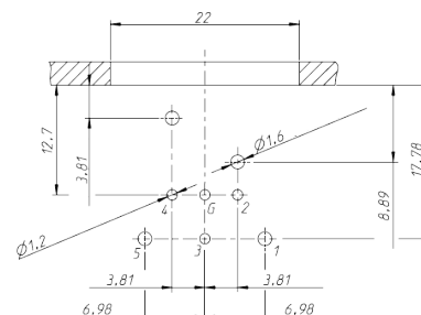
Макет печатной платы. Вид со стороны установки PCB layout. Component side
