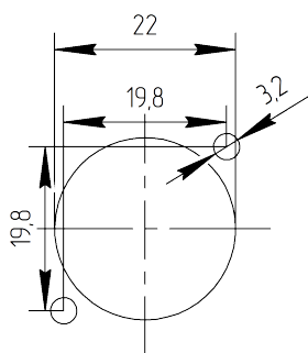
Монтажное отверстие. Вид сзади Cut out dimensions. Rear view
