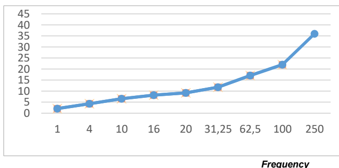
Attenuation
