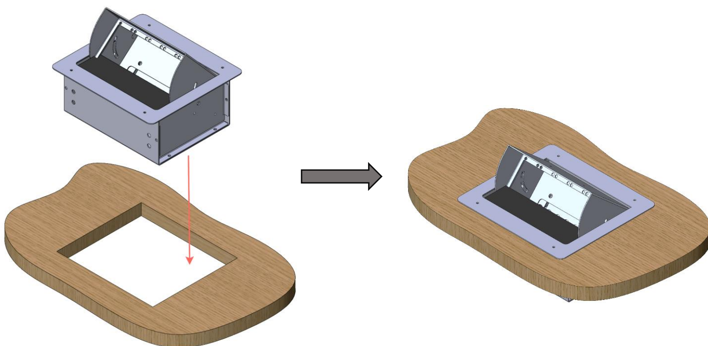
Рис.2 Установка лючка в стол
