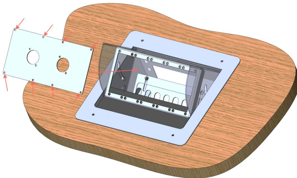
Рис. 3. Установка панели в бокс лючка
