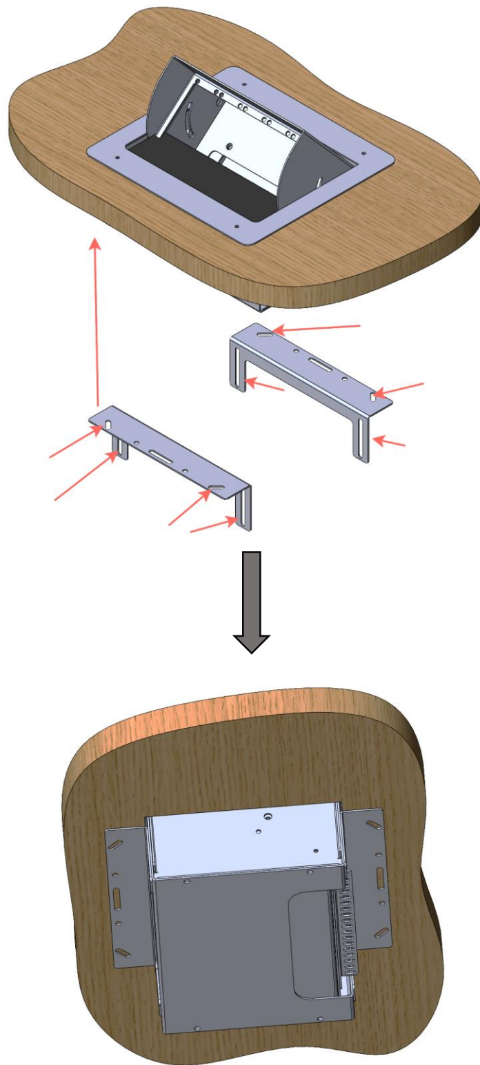
Рис. 5. Крепление лючка к столу при помощи уголков
